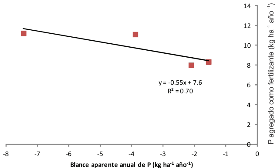
Figura 4. Relación entre fósforo agregado como fertilizante a los cultivos y el balance aparente anual de fósforo (EEMAC, período 2001-2010).
