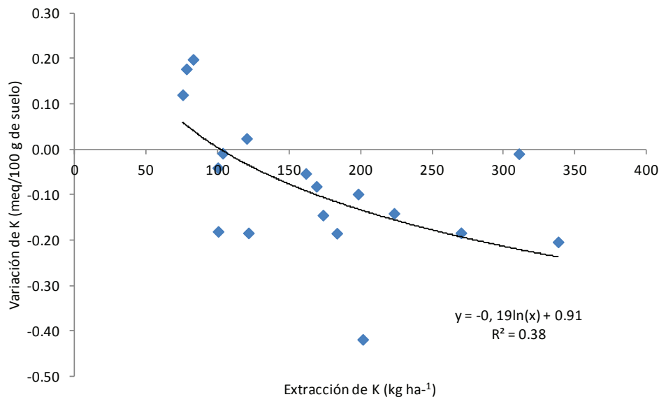
Figura 5. Relación entre la variación de potasio (meq/100g) y la extracción (kg ha -1 ) en los primeros 10 cm el perfil de suelo.
