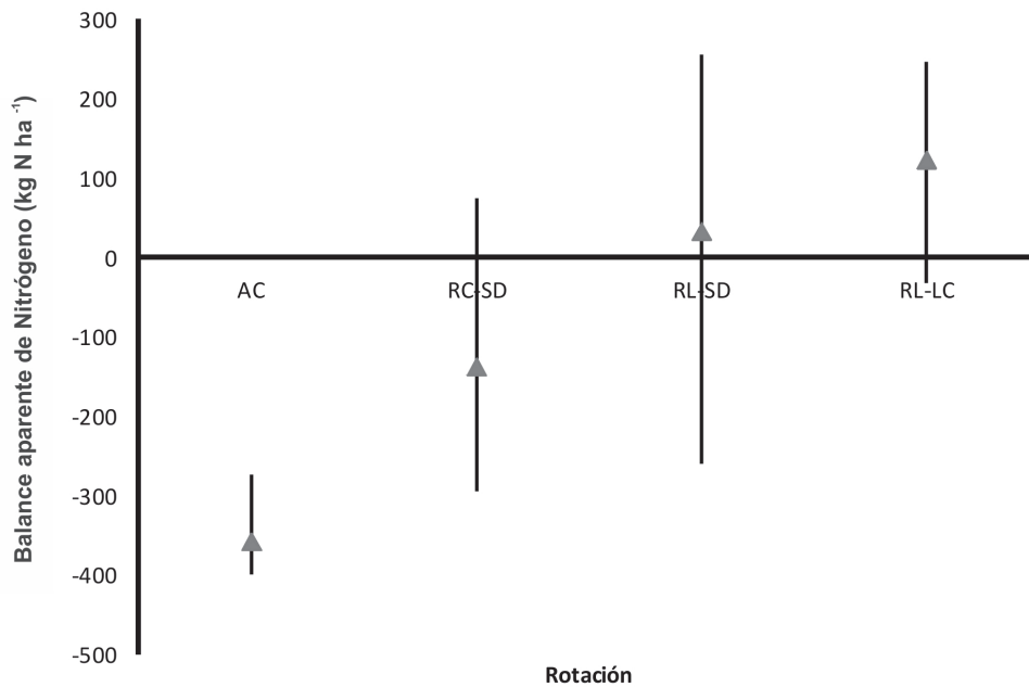
Figura 1. Balance medio acumulado de nitrógeno, mínimo y máximo cuantificado a abril 2011 según los tratamientos agricultura continua (AC), rotación corta con pasturas (RC-SD), rotación larga con pasturas (RL-SD) y rotación larga con pasturas con laboreo convencional (RL-LC) en kg ha -1 .
