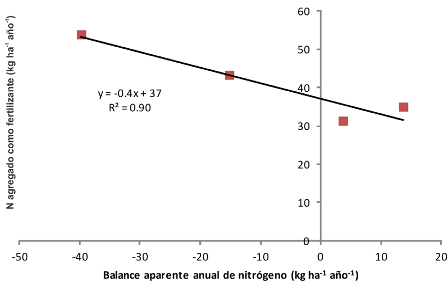
Figura 2. Relación entre nitrógeno agregado como fertilizante a los cultivos y el balance aparente anual de nitrógeno (EEMAC, período 2001-2010).
