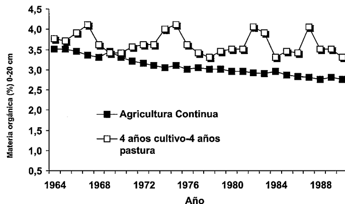
Figura 1. Contenido de materia orgánica del suelo desde 1964 hasta 1990, en sistemas agrícolas continuos o en sistemas agrícolas en rotación con pasturas, ambos con laboreo convencional (Tomado de Díaz Roselló, 1992).
