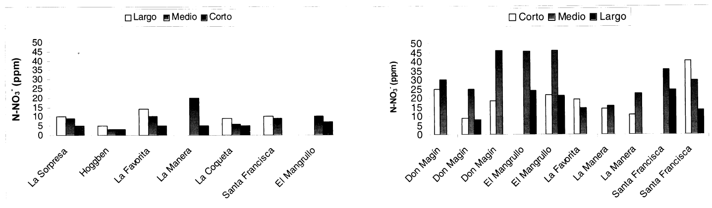
Figura 2. Disponibilidad de N-NO 3 - en el suelo (0 - 20 cm) a la siembra en respuesta al tiempo de barbecho en dos años con lluvias contrastantes.
