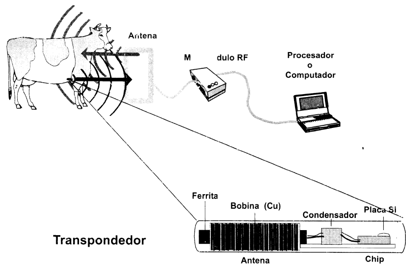
Figura 1. Esquema de los principales componentes de un sistema de identificación electrónica por radiofrecuencia.
