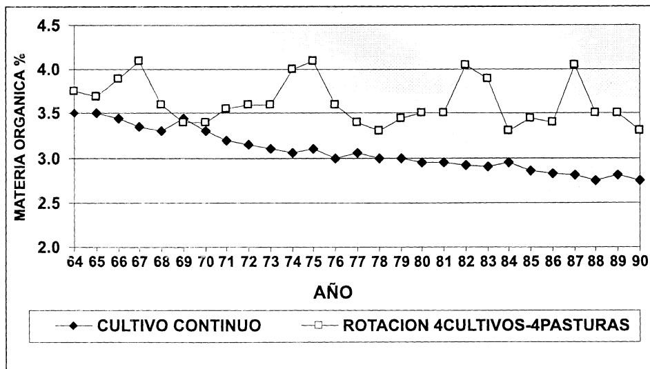
Figura 4. Consecuencias de las rotaciones sobre la calidad del suelo (Díaz, 1992).
