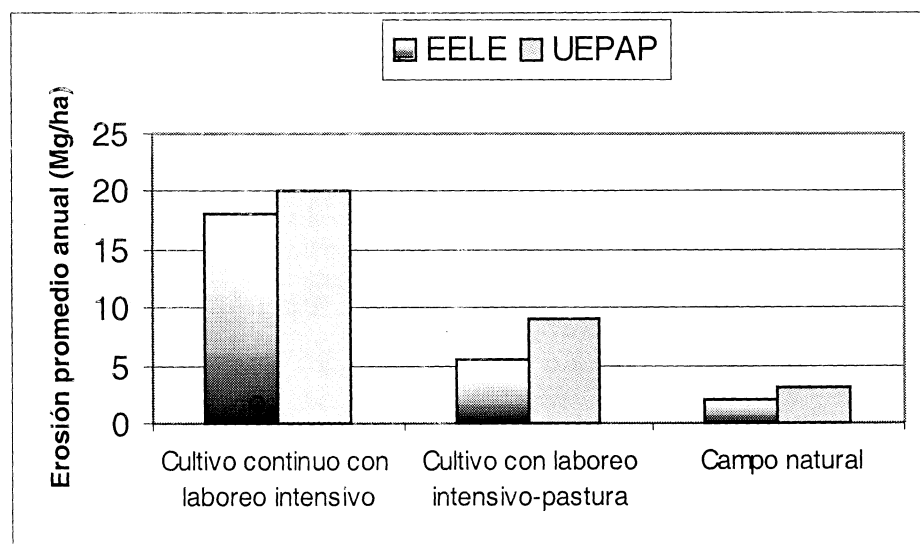
Figura 6. Consecuencias de las rotaciones sobre la erosión: parcelas de escurrimiento en La Estanzuela (EELE, 1984 - 1990, Sawchik y Quintana, cit. por García Préchac, 1992b) y en Palo a Pique (UEPAP, 1993 - 1999, Terra y García Préchac, 2001).
