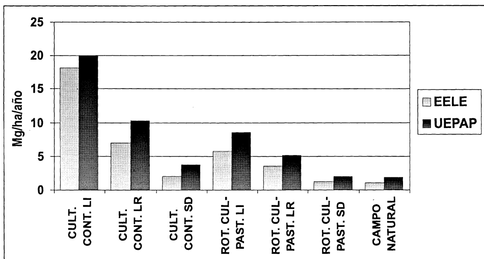
Figura 12. Erosión promedio anual en parcelas de escurrimiento, llevadas a 100 m de pendiente. EELE: 1984 - 1990, Sawchick y Quintana, citados García Préchac (1992b); UEPAP: 1994 - 1999, Terra y García Préchac, 2001.
